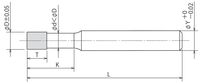
φDの公差は#100～#1000選択時に適用。
